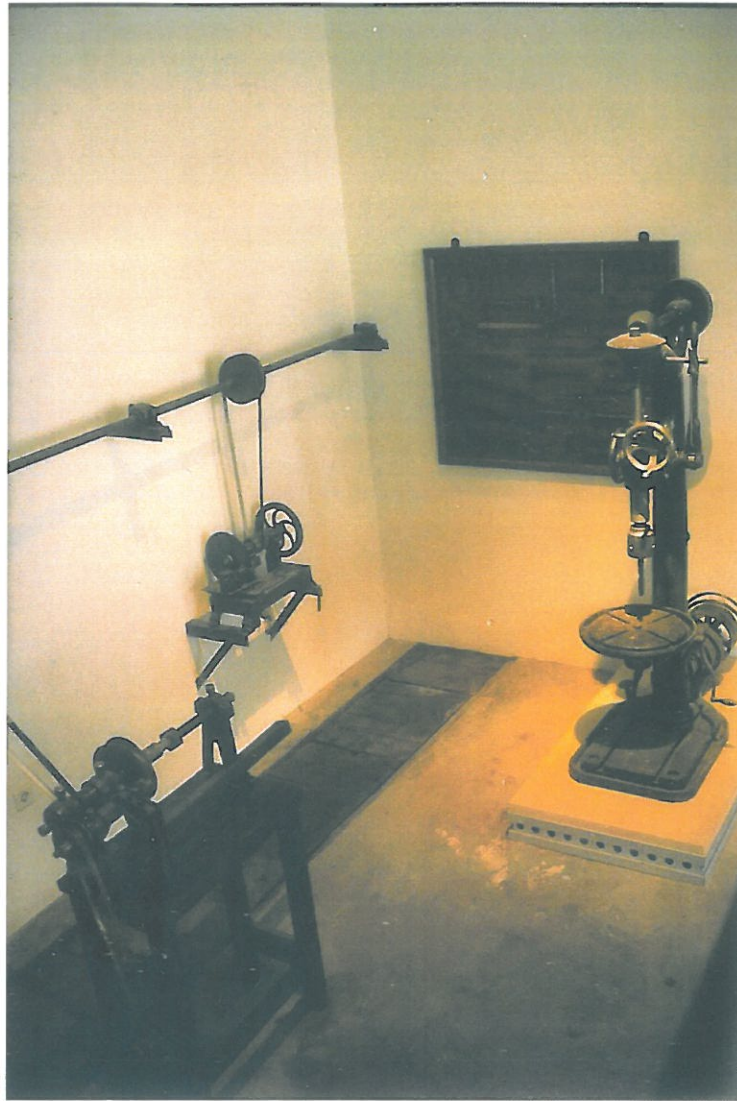
Oficina de Serralharia. Reconstituição museológica do posicionamento das máquinas-ferramentas.
